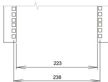
10" SYSTEM – WYMIARY
