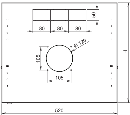
GÓRNY WIDOK
