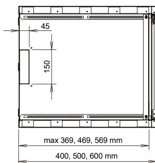
POKRYWA GŁĘBOKOŚĆ 500 MM
